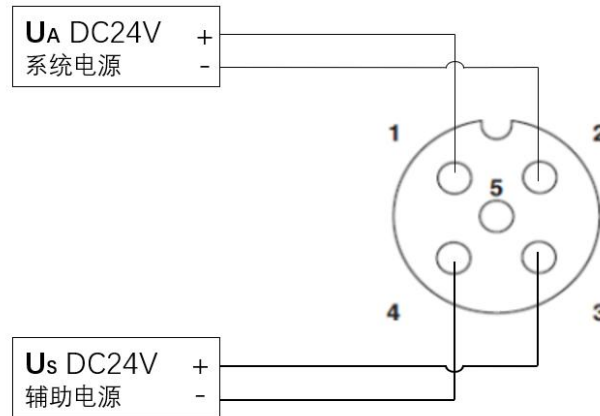
电源接口
