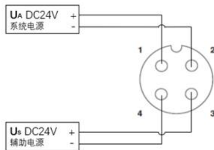
电源端口
